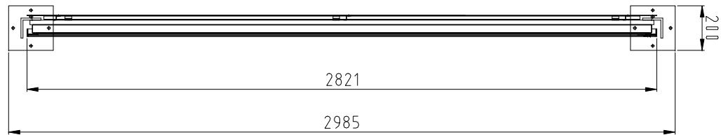
Leuchtkasten F12 freistehend, einseitig
